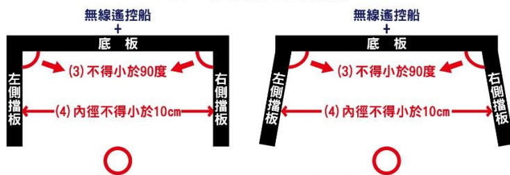
圖2、推球板示意圖(俯視)
